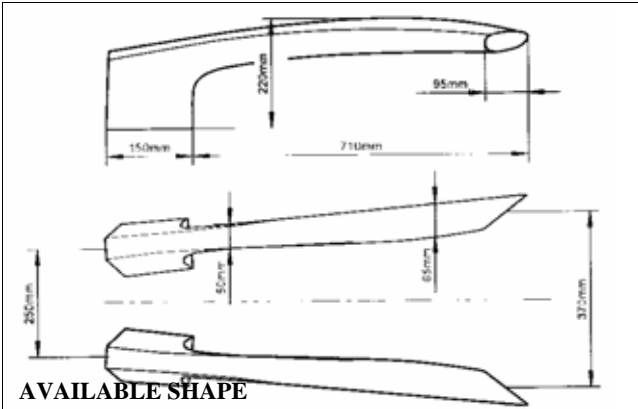
模具示意图
